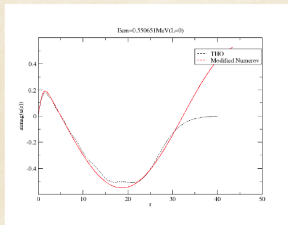
Figure 6.176: L = 0 的波函数虚部的符合情况
