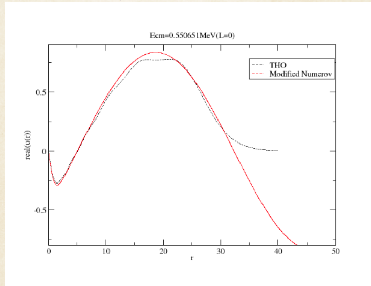
Figure 6.175: L = 0 的波函数实部的符合情况
